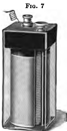
FIG. 7 Wet Leclanché cell.
